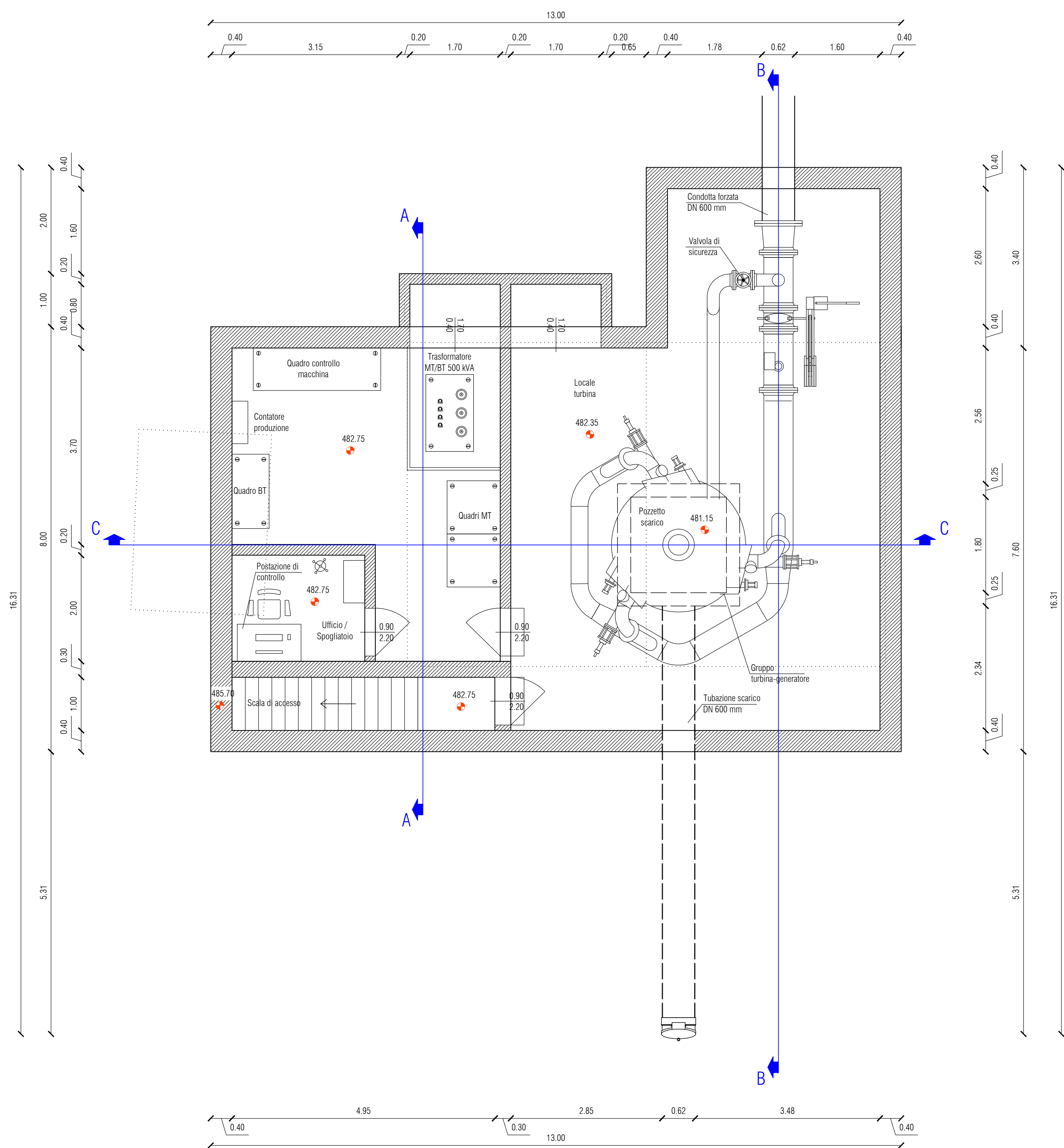
PIANTA CENTRALE PIANO -1 Scala (1:50)
