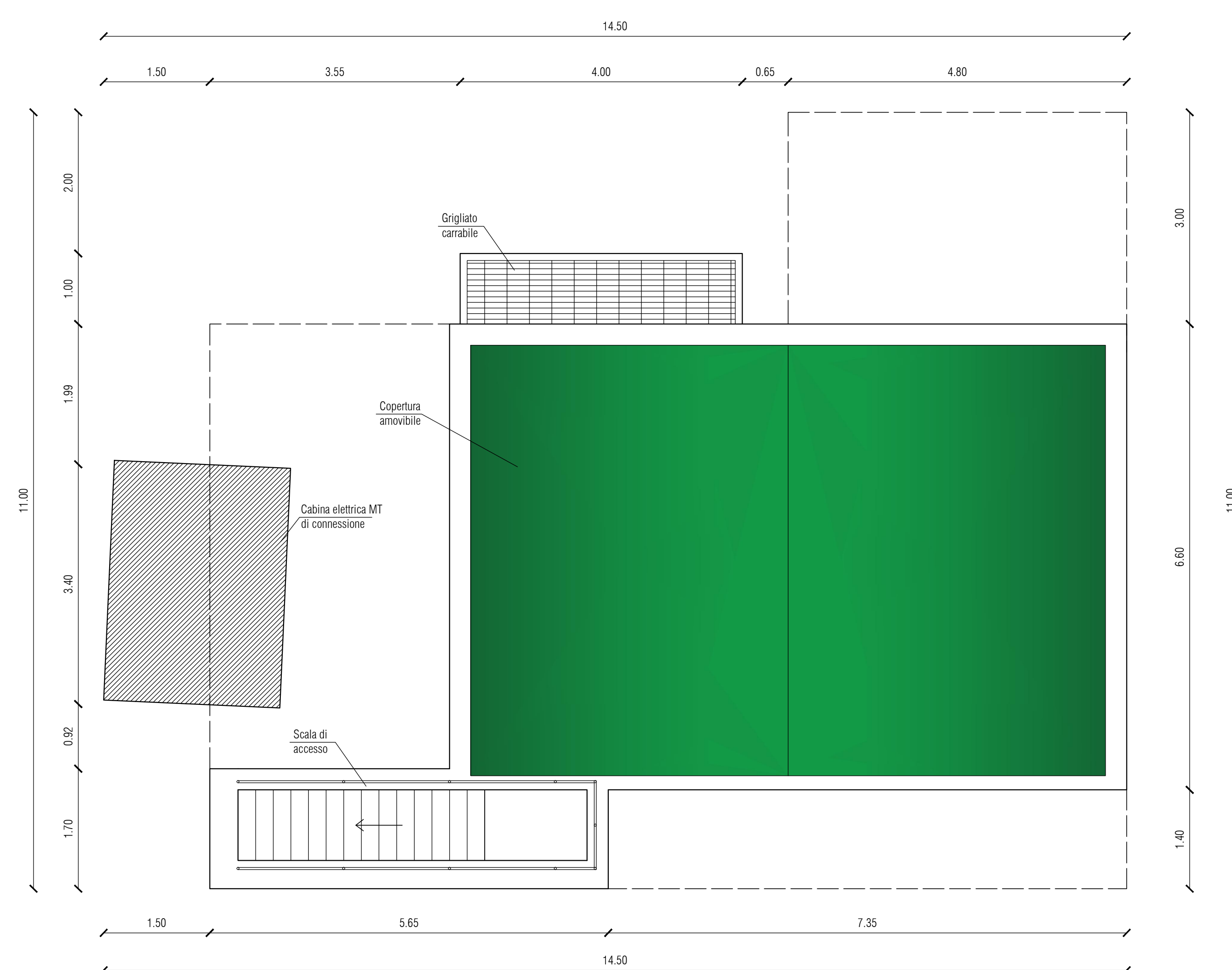
PIANTA CENTRALE PIANO CAMPAGNA Scala (1:50)
